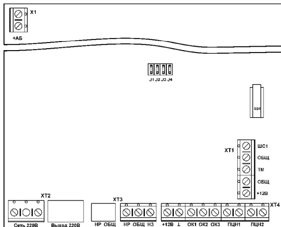
Рис. 1 Плата контроллера
