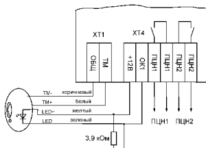
Рис. 7 Схема подключения ПЦН и порта Touch Memory
