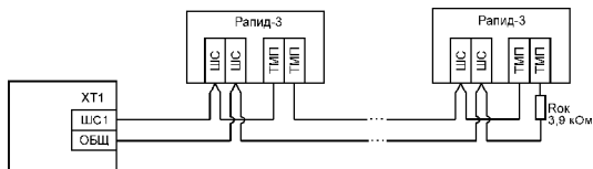
Рис. 4 Схема внешних соединений в охранных режимах (* устанавливается на извещателе двери для задержки звукового сигнала в тактиках «Централизованная охрана 2» и «Ведомственная охрана»)
