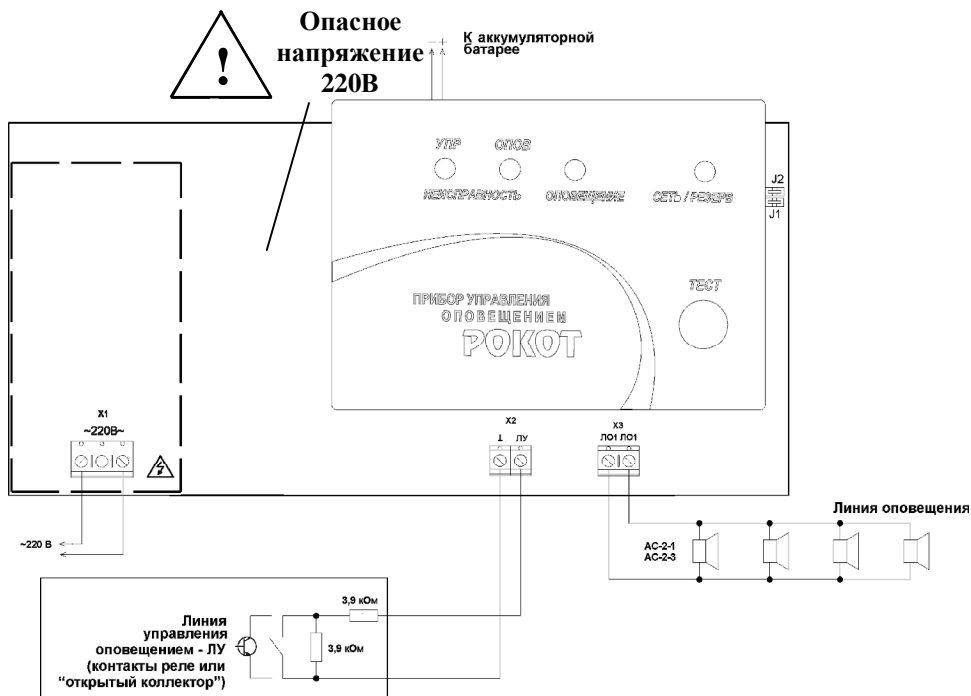
Рис. 1 Схема подключения прибора «Рокот»
