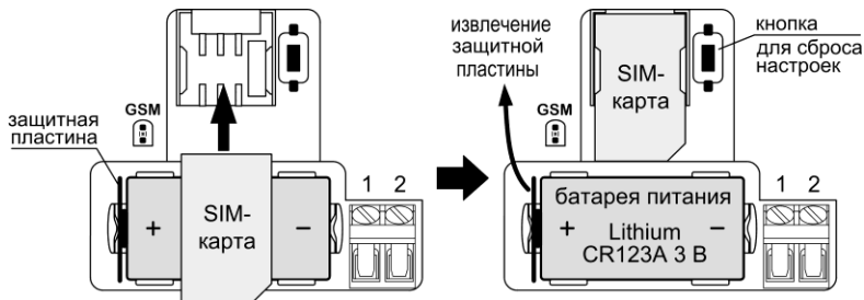
Рис.3 Установка SIM-карты, включение питания - извлечение защитной пластины
