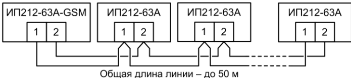
Рис.6 Схема соединения извещателей в группу
