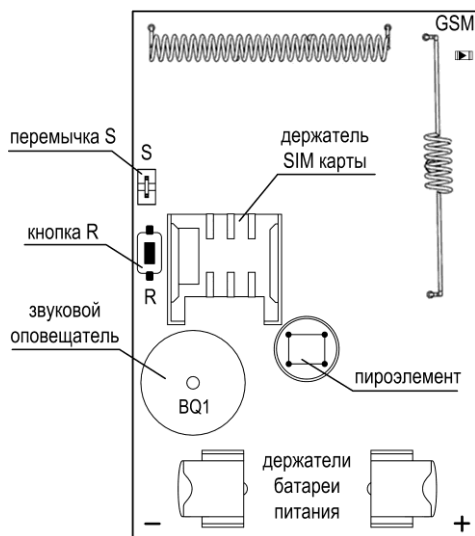
Рис.2 Плата сигнализатора
