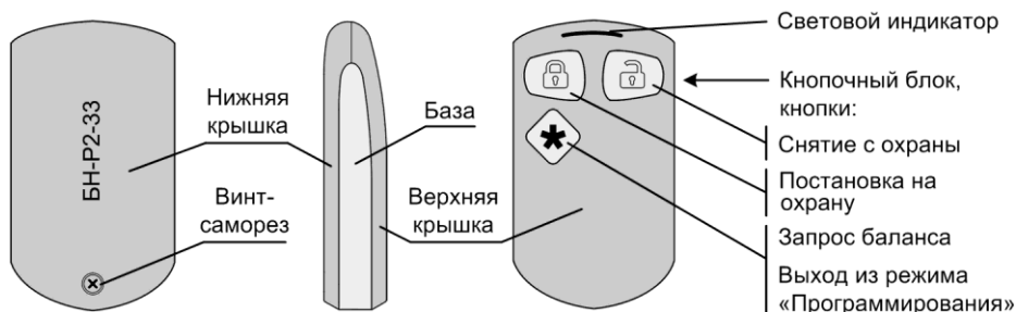
Рис.3 Конструкция брелока. Общий вид
