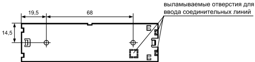
Рис.6 Присоединительные размеры
