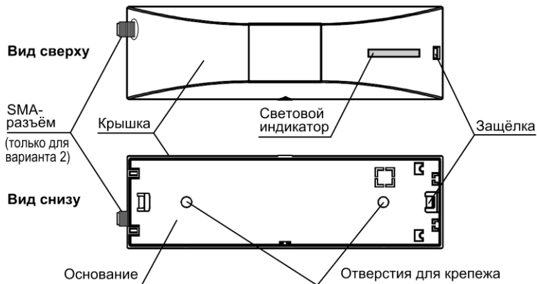
Рис.1 Конструкция сигнализатора. Вид сверху и снизу
