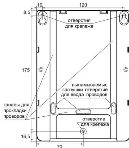
Рис.2 Присоединительные размеры
