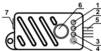
Рис.1 Внешний вид программатора
