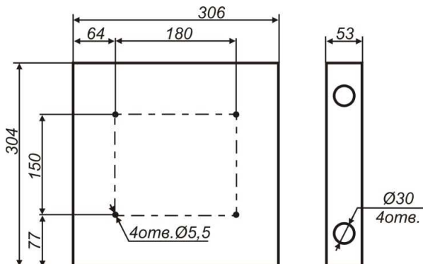
Габаритные и присоединительные размеры шкафа для УВКП
